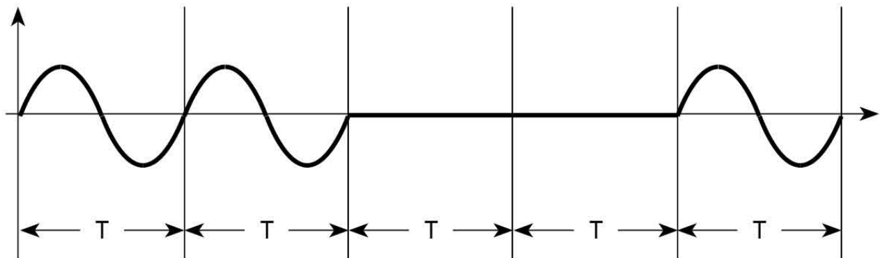
Рисунок 4.15. Форма выходного сигнала в режиме «Субгармоники» (T — период сигнала)
